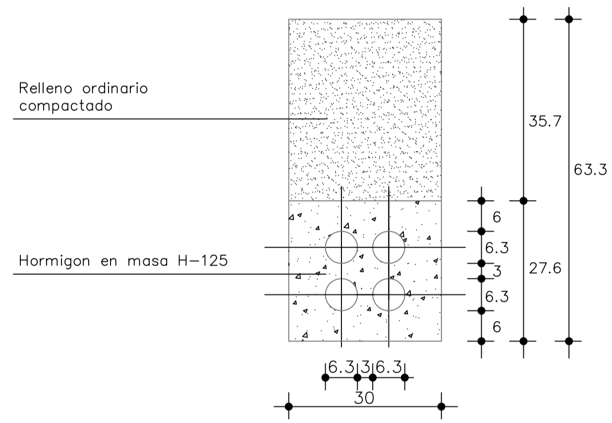
CUATRO CONDUCCIONES DE 63 mm \phi
