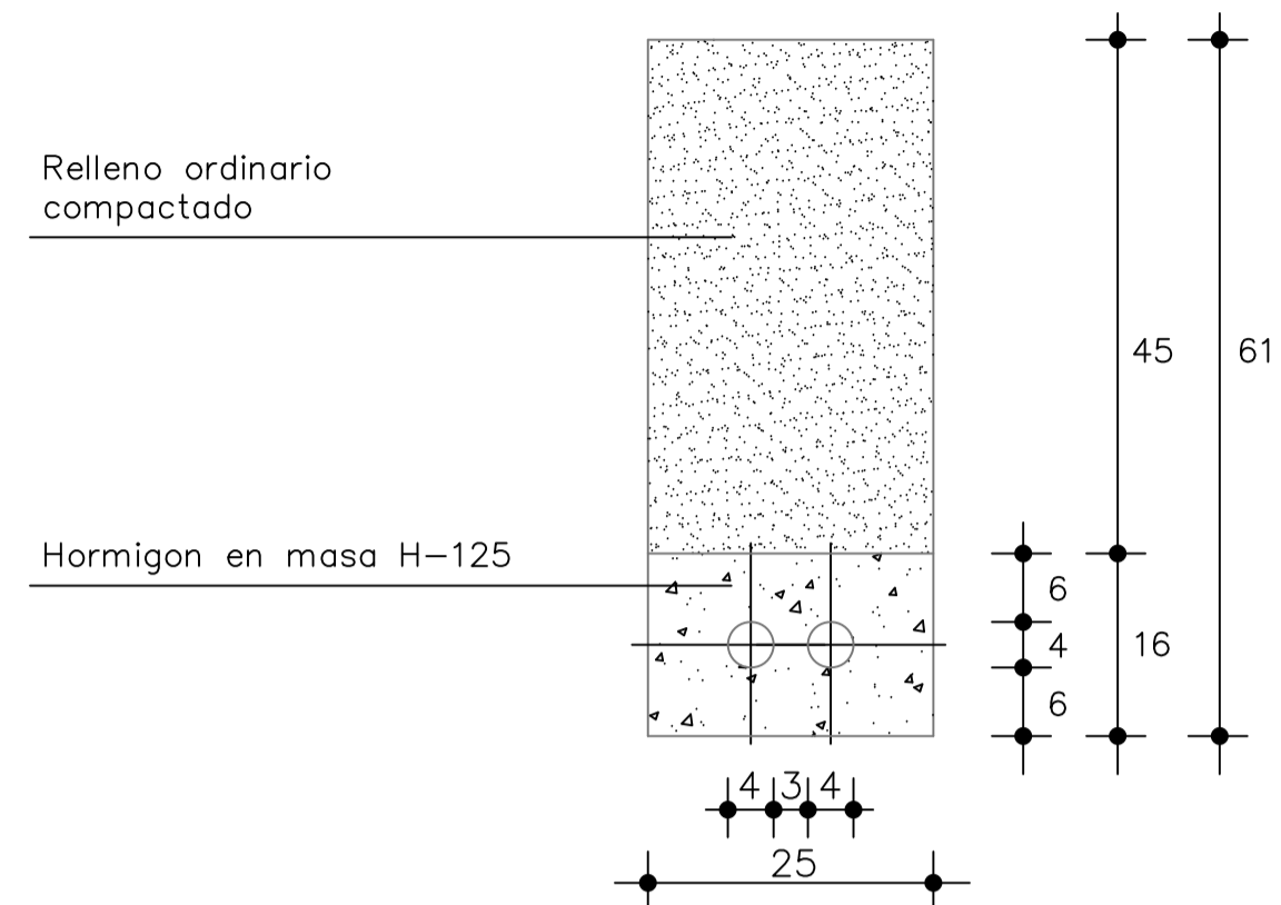
DOS CONDUCCIONES DE 40 mm \phi
