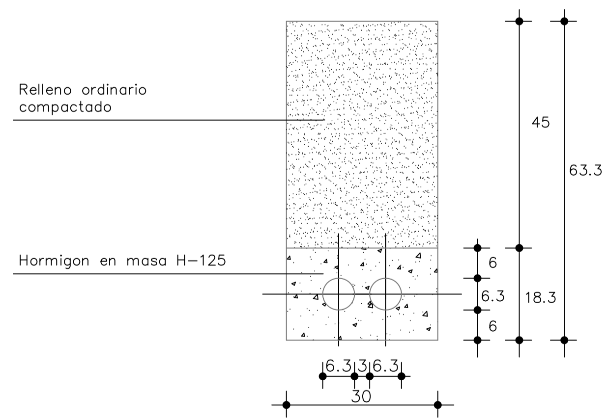
DOS CONDUCCIONES DE 63 mm \phi
