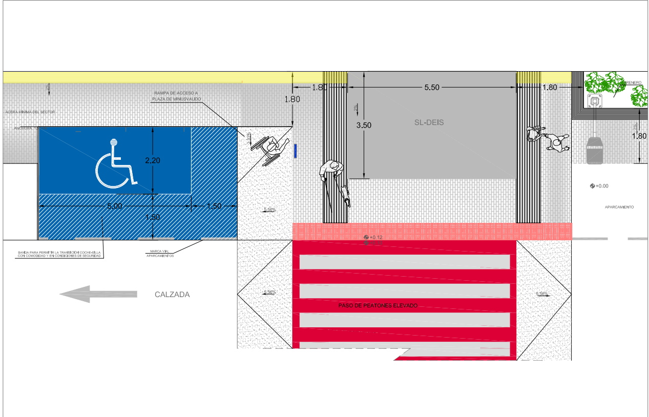
APARCAMIENTO RESERVADO PARA PERSONAS CON MOVILIDAD REDUCIDA. ESQUEMA
